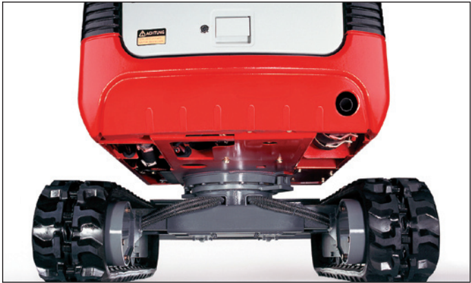
Gran distancia del eje al suelo, cárter del motor cerrado y protegido y ancho de vía hidráulicamente variable
