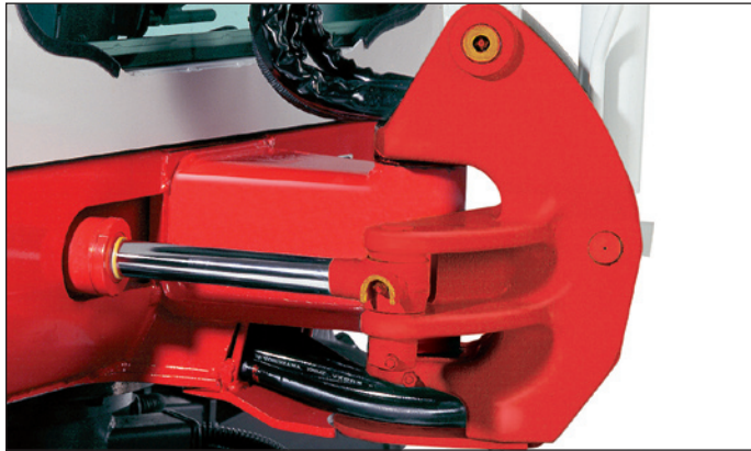
Bloque de giro del brazo robusto con latiguillos protegidos con giro hidráulico del brazo
